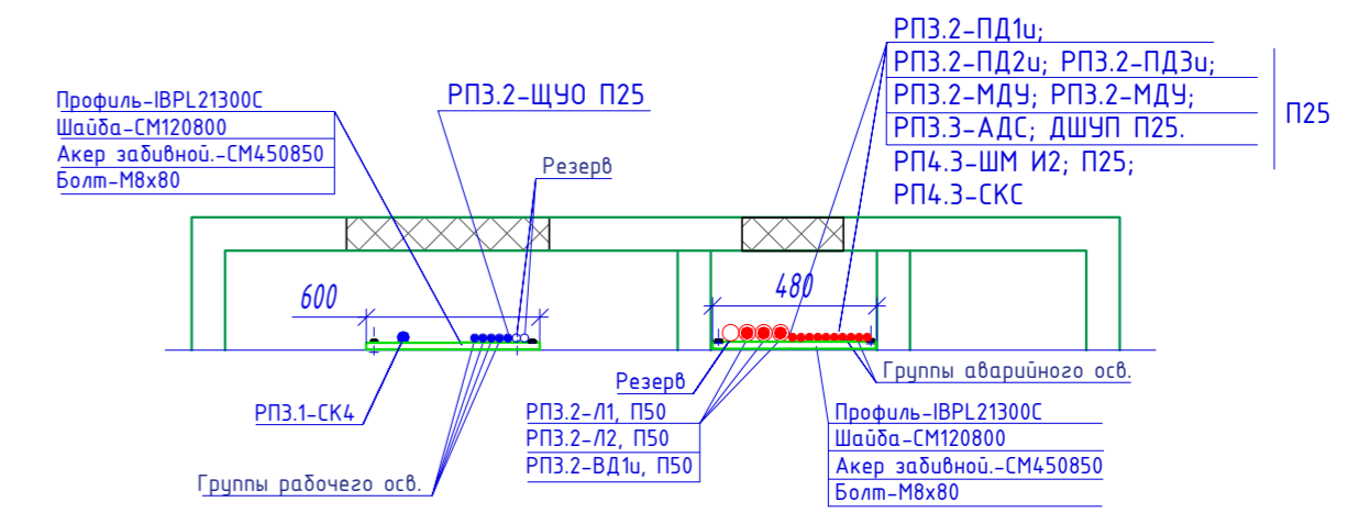
Фрагмент 1 Крепление кабеля в электротехнической нише
